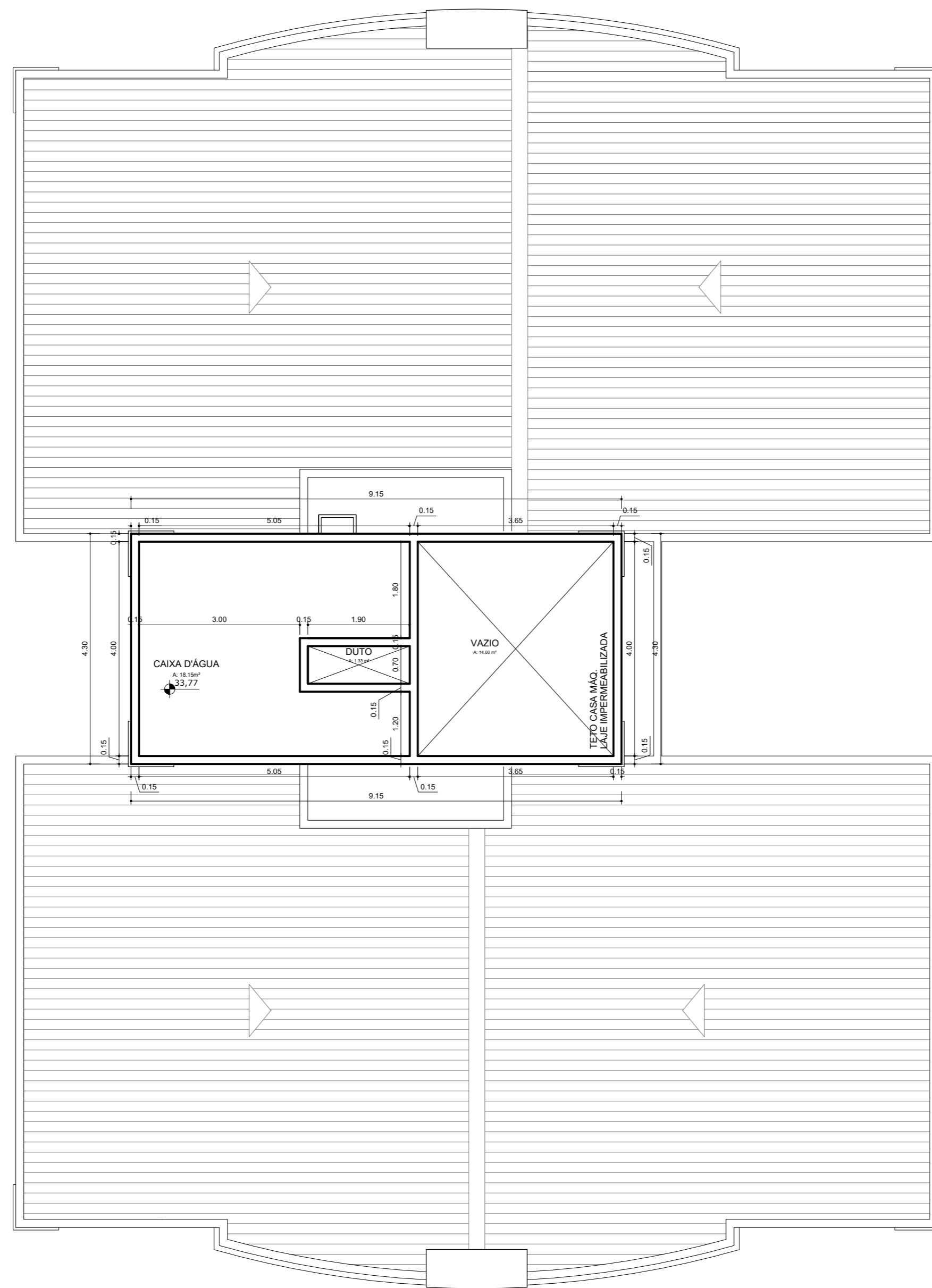
PLANTA BAIXA PAVTO CAIXA D'ÁGUA - TORRE01/ 02/ 07/ 08/ 09 ÁREA DO PAVTO: 24,74 m²
